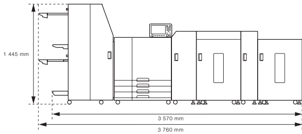
Alimentation et réception double haute capacité 2 x 4 000 feuilles
